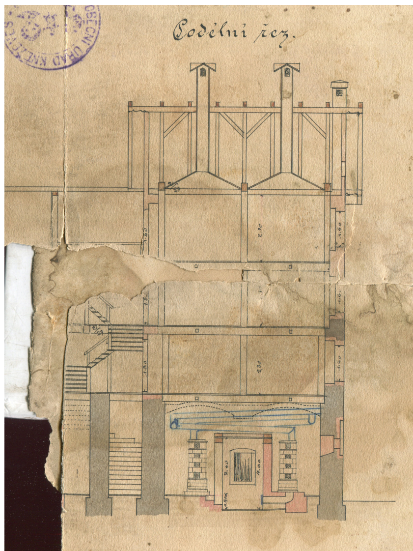
Průřez sušárnou v čp. 102
