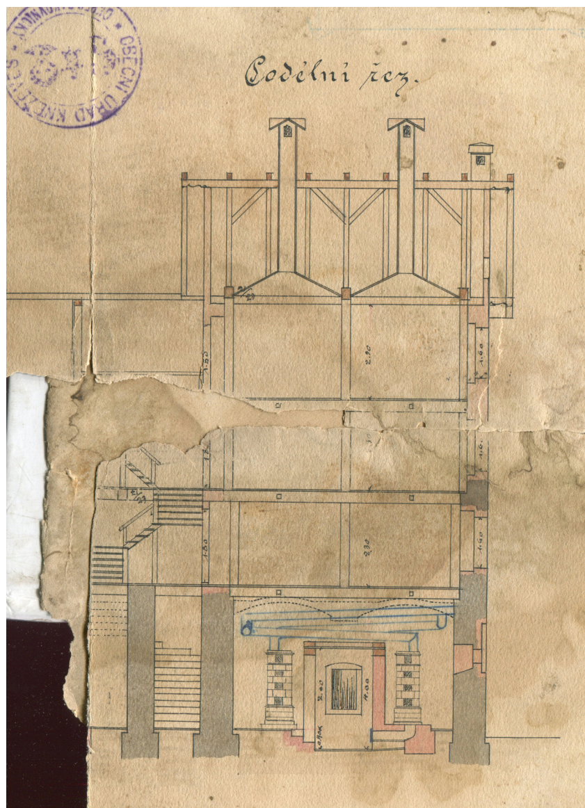
Průřez sušárnou v čp. 102
